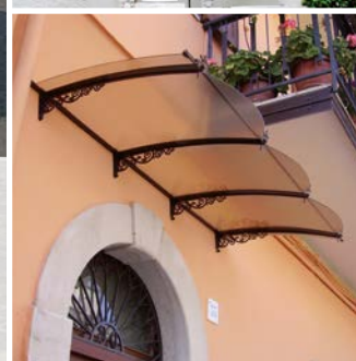
Pensilina LIBERTY Mod. LT-01 Larghezza 2,30, sporgenza 1,30 Struttura: Antracite P016V Grinz Copertura: Neutro satinato
