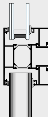
Sottotraversi di finestre in Alluminio e PVC
