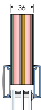
Tipo TP 36 Up 0.86 W/m 2 k Rw 33 dB Kg 20,0 m 2
