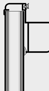
Scuri esterni con telaio a scomparsa
