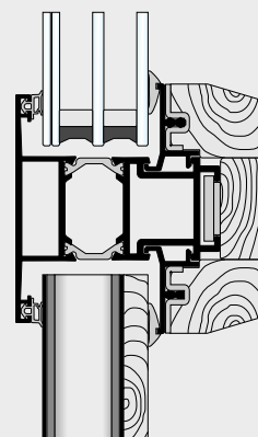
Sottotraversi di finestre interno Legno
