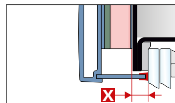
Particolare aletta cingivetro su pannelli a vetri delle collezioni A Filo e Emotion .
