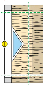
Fig. 2 area decorativa vincolata ai lati
