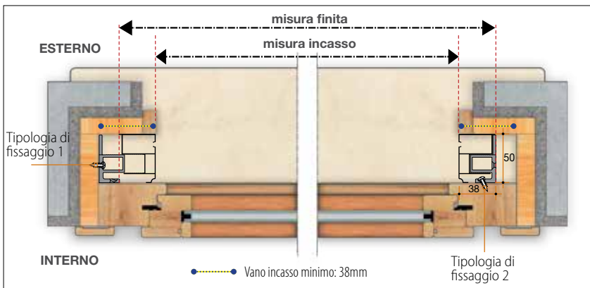
Sezione orizzontale
