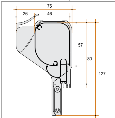
Cassonetto con barra maniglia e cuffia Clever
