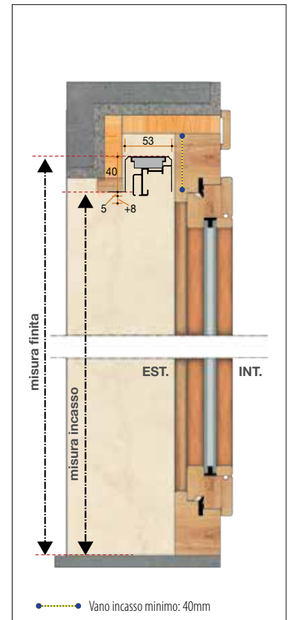
Sezione verticale
