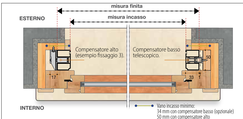
Sezione orizzontale
