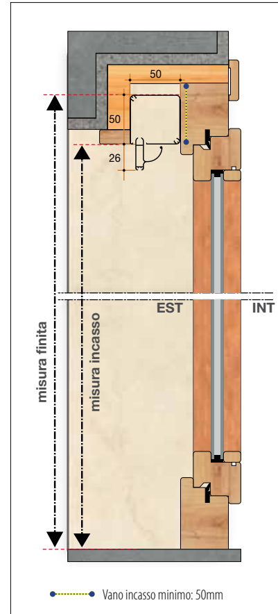
Sezione verticale
