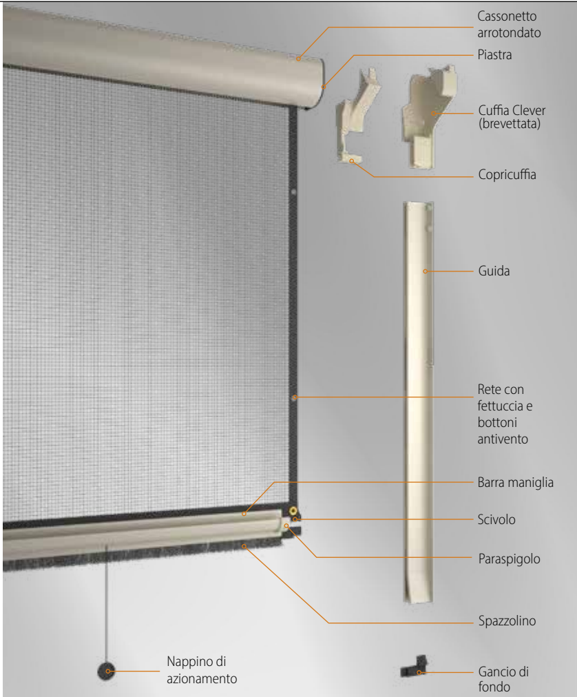
Cuffia Clever (brevetto internazionale Bettio)
